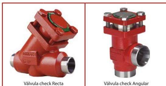
Válvula check Recta
